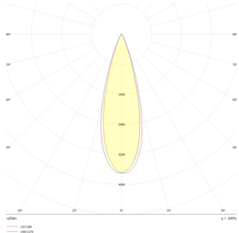
Magnetrack Pro Suspendido 7W 24°
