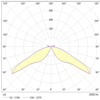
Miniposte 18W 130°
