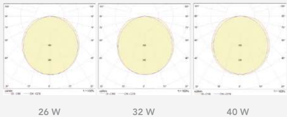
FOTOMETRÍA
