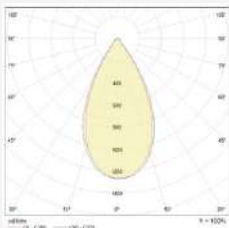
AC1410 Óptica 55°
