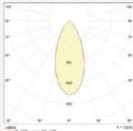
42 W : 60°
