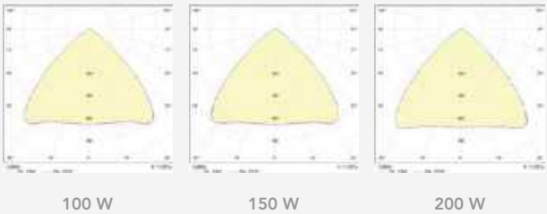
FOTOMETRÍA
