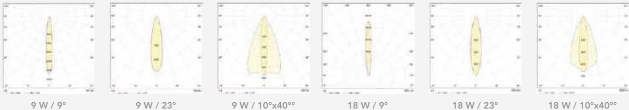
FOTOMETRÍA
